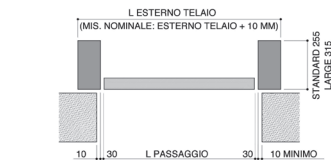
POSIZIONE OLTRE LUCE STRUTTURA SIKURTEC CITY HF
