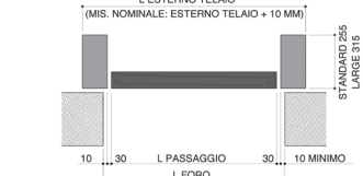
POSIZIONE OLTRE LUCE STRUTTURA SIKURA CITY HF
