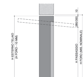
POSIZIONE IN LUCE STRUTTURA SIKURA HF
