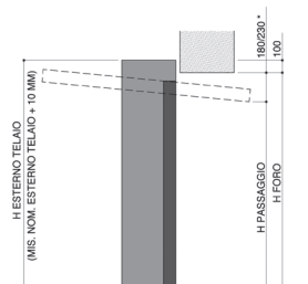
POSIZIONE OLTRE LUCE STRUTTURA SIKURTEC HF
