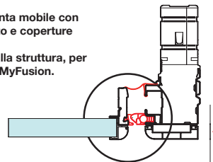
POSIZIONE IN LUCE STRUTTURA SIKURTEC CITY HF
