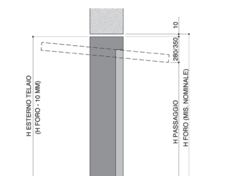
POSIZIONE IN LUCE STRUTTURA SIKURA HF
