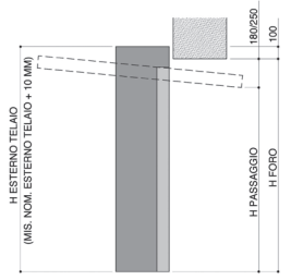
POSIZIONE OLTRE LUCE STRUTTURA SIKURA HF
