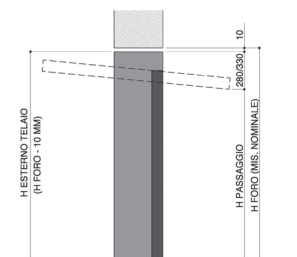
POSIZIONE IN LUCE STRUTTURA SIKURTEC HF
