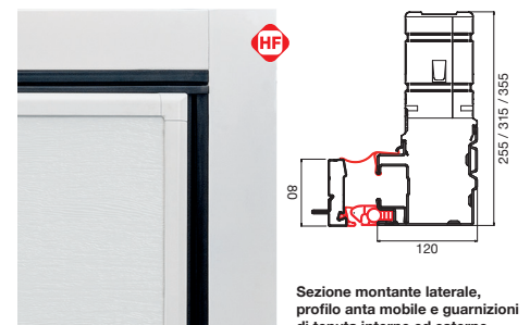
Sezione montante laterale, profilo anta mobile e guarnizioni di tenuta interne ed esterne.
