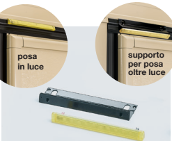
Lampeggiante a led esterno, con antenna integrata, montato e precabato, posto a sinistra in esterno sulla traversa superiore. (cod. MB.10.01) (optional)
