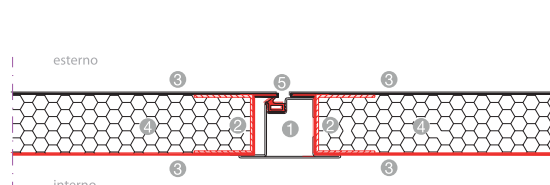
Particolare inversione di battuta Pronta
