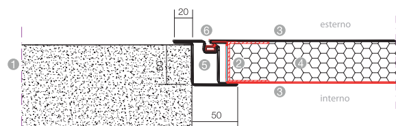
Particolare cassa-anta Pronta
