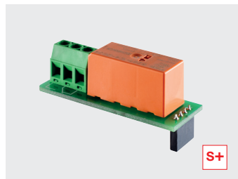
Relè extra, per accendere l'illuminazione esterna/interna insieme all'automazione. Disponibile solo per automazioni S+ green . (cod. SZ950) (optional)
