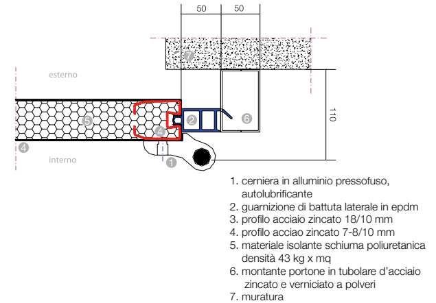
Particolare incontro di battuta oltre luce
