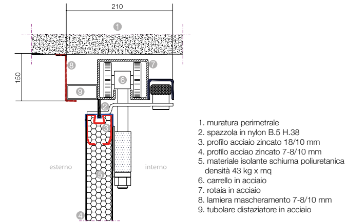
Particolare superiore ANTEO montato in luce
