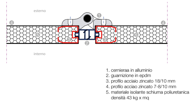
Particolare cerniera tra anta e anta
