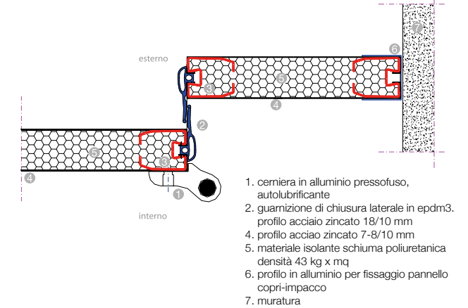
Particolare chiusura laterale in luce con pannello copri-impacco
