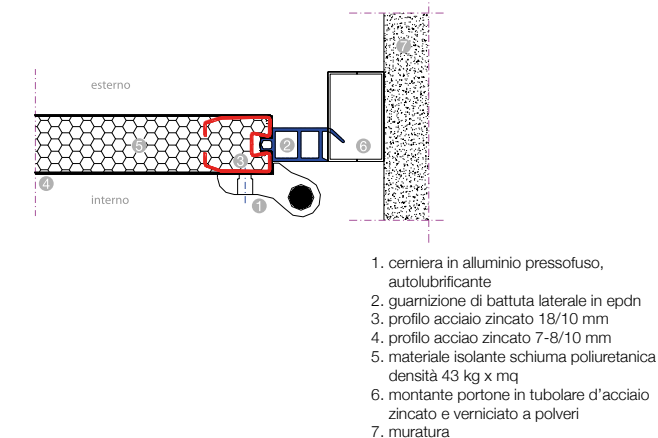
Particolare incontro di battuta in luce
