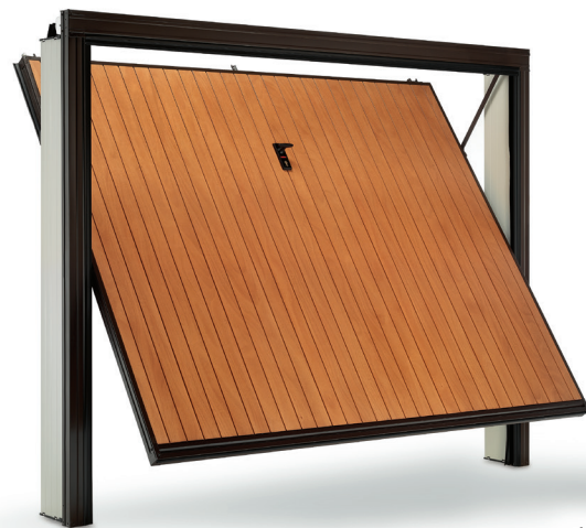
Porta basculante Slide Spazio HF, rivestimento esterno in Okoumé multistrato pantografato a doghe verticali, passo da 85 mm. La predisposizione alla motorizzazione HF, il trattamento completo in tinta 1 e la guarnizione inferiore in gomma sono optional.
