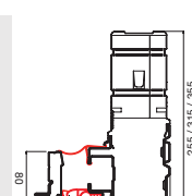
Sezione montante laterale, profilo anta mobile e guarnizioni di tenuta interne ed esterne.
