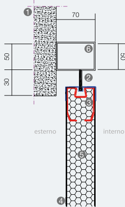
Particolare superiore portone ALISEO montato oltre luce
