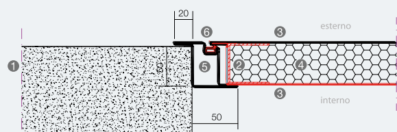
Particolare cassa-anta Pronta
