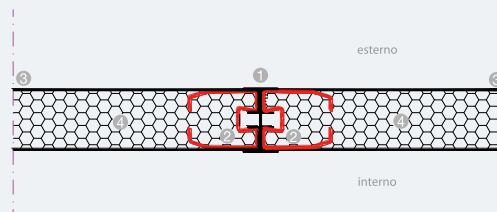
Particolare giunzione pannelli
