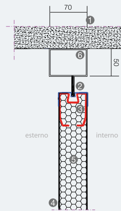
Particolare superiore portone ALISEO montato in luce
