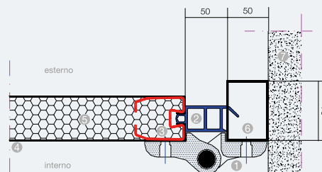
Particolare laterale di chiusura in luce
