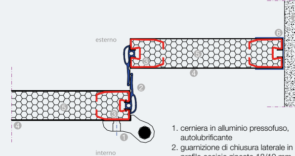
Particolare chiusura laterale in luce con pannello copri-impacco
