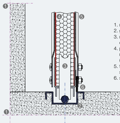
Particolare inferiore portone ROTEO GOLD con guida incassata
