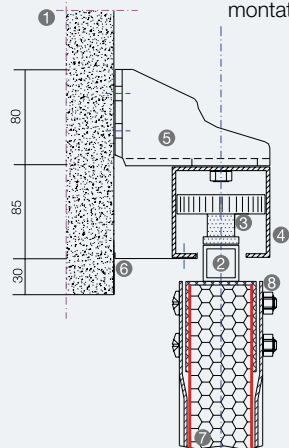
Particolare inferiore portone ROTEO GOLD con guida inferiore ad omega
