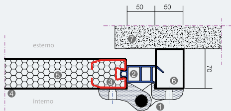
Particolare laterale applicato oltre luce
