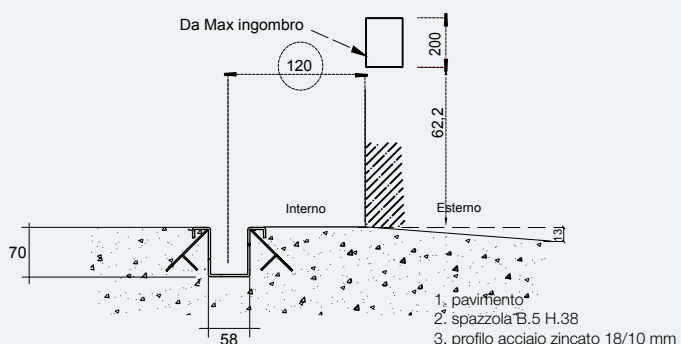
Particolare inferiore montato oltre luce interno
