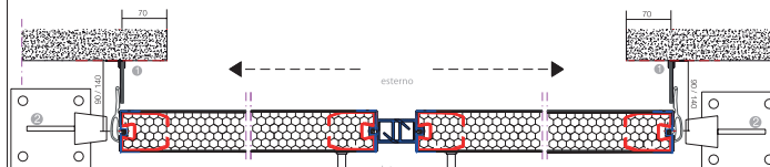
Particolare inferiore ROTEO GOLD montato oltre luce a due ante, asse 90 / 140 mm
