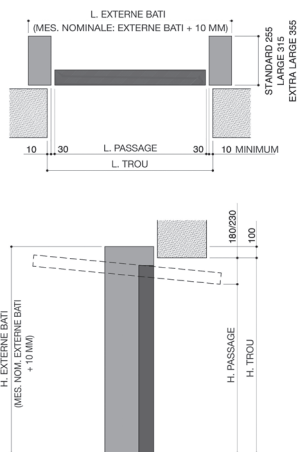
POSITION EN APPLIQUE STRUCTURE SIKURA HF
