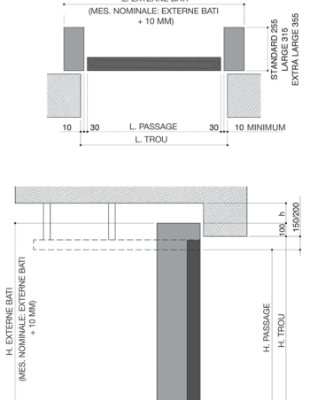
POSITION EN APPLIQUE STRUCTURE SIKURA CITY HF
