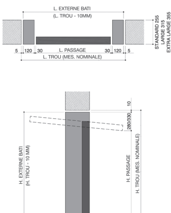
POSITION EN TUNNEL STRUCTURE SIKURA HF
