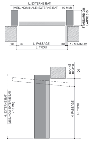
POSITION EN APPLIQUE STRUCTURE SIKURTEC HF
