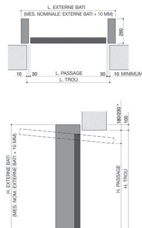
POSITION EN APPLIQUE STRUCTURE SPAZIO HF
