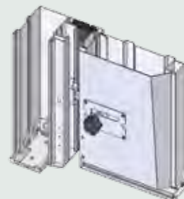
Catenaccioli laterali interni per anta mobile porta basculante con automazione.
