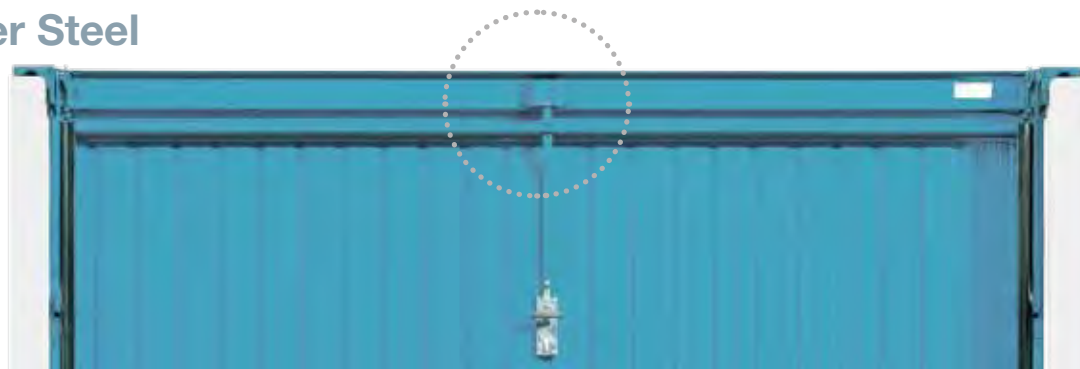
Vista interna serratura standard a 1 punto di chiusura centrale per strutture Spazio, Spazio HF, Sikurtec, Sikurtec HF, Sikurtec HF City e Sikura (manuale).
