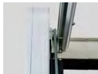
Particolare degli spazi di sicurezza ottenuti tramite la predisposizione HF.
