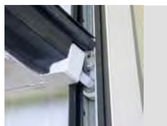
Dispositivo paracadute inserito nelle guide. Agisce in caso di rottura delle funi bloccando la caduta dell'anta mobile.
