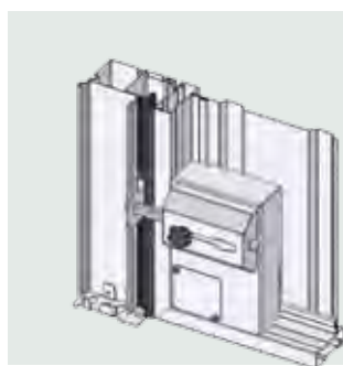
Catenaccioli manuali laterali interni per anta mobile con struttura Spazio, Sikurtec, Sikurtec City, Sikura e Sikura City.
